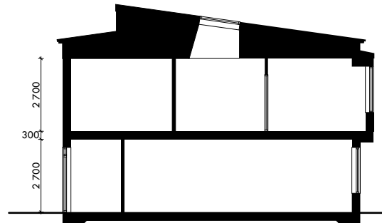
TYPSEKTION
